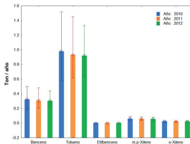
Figura 1. Resultados de las emisiones anuales de COV al ambiente por la presencia de gasolineras en la zona urbana
